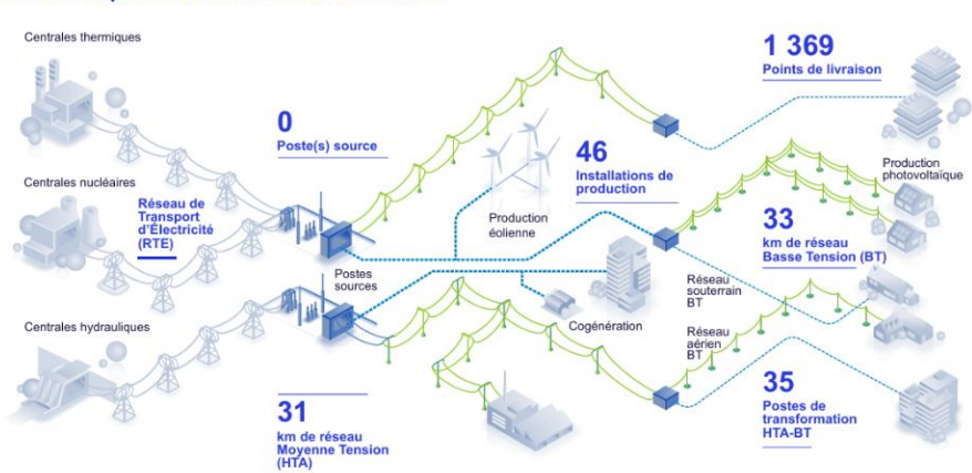
Le réseau public de distribution d'électricité
